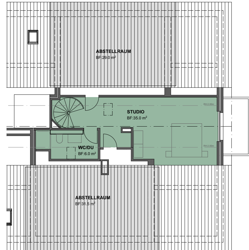
2. DACHGESCHOSS
