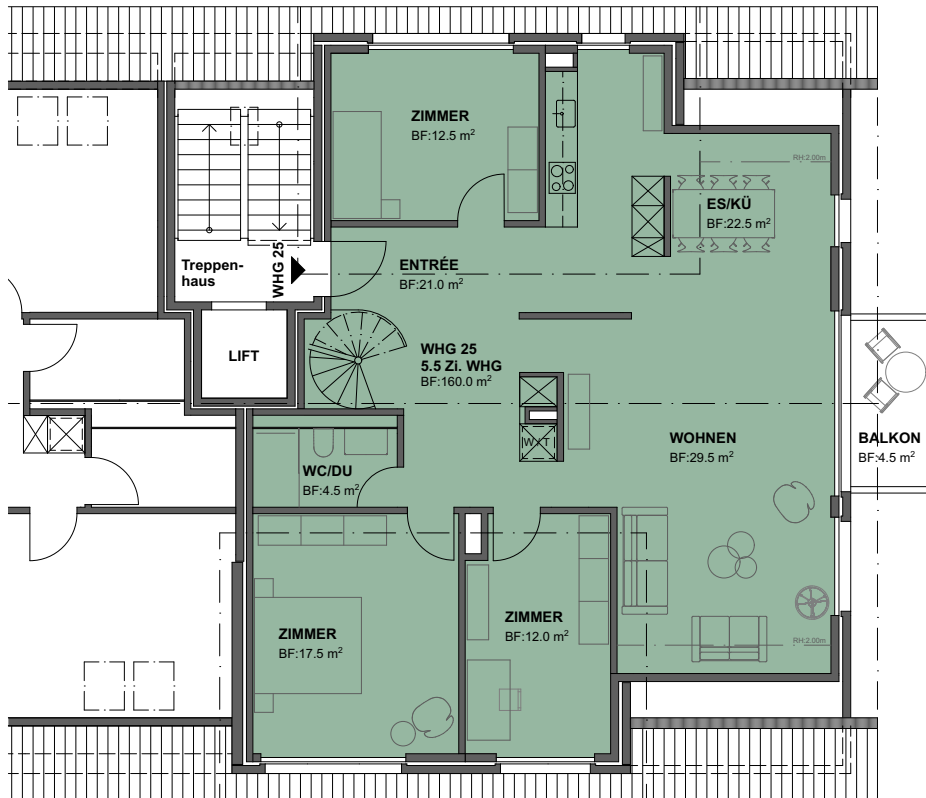
1. DACHGESCHOSS
